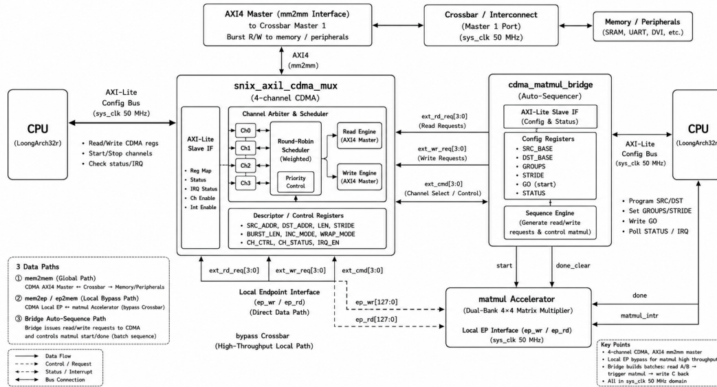
图 2: DMA/CDMA 数据搬运子系统架构
