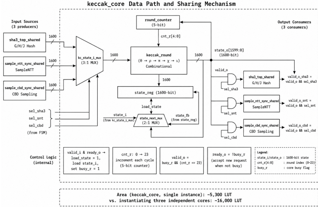
图 3: Keccak-f[1600] 核数据通路与共享机制
