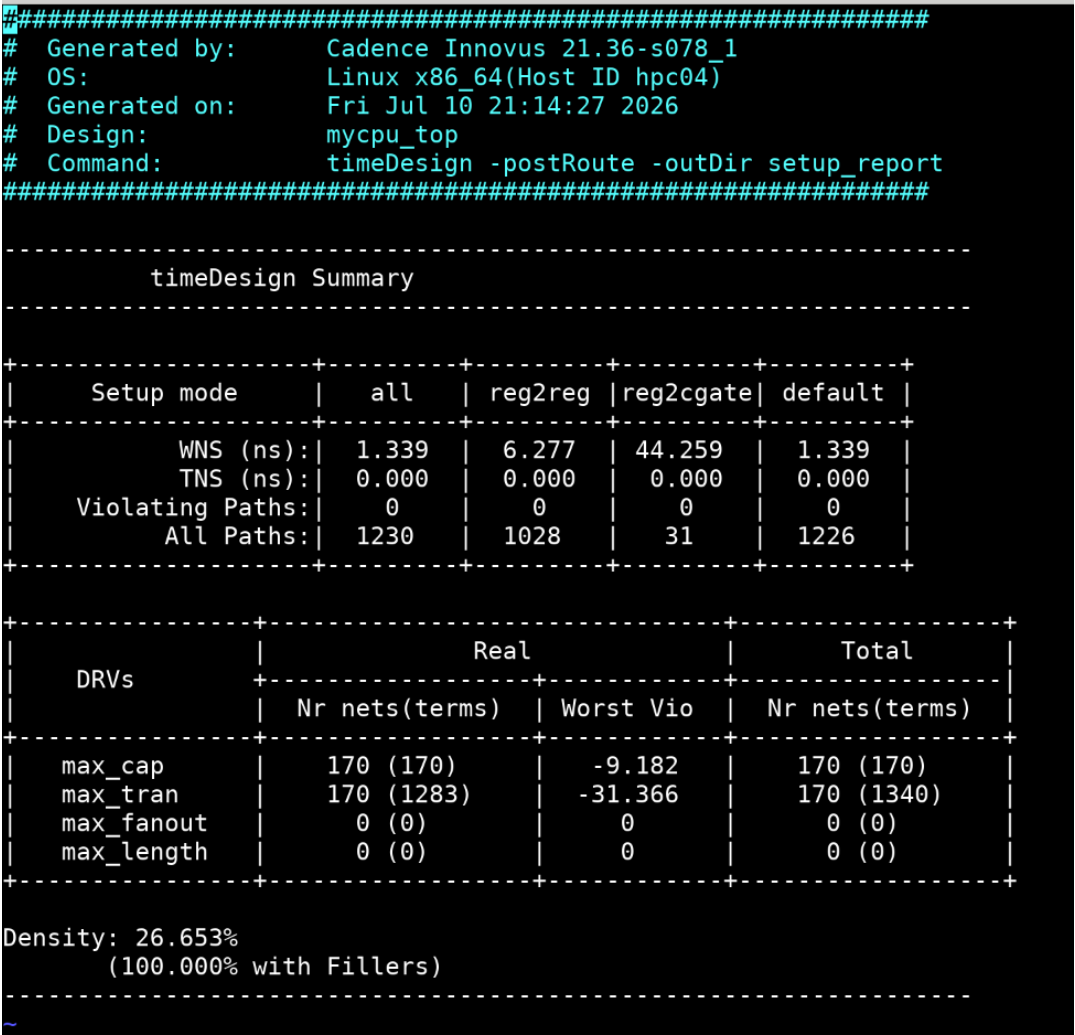
图 8: 建立时间 (Setup) 时序汇总
